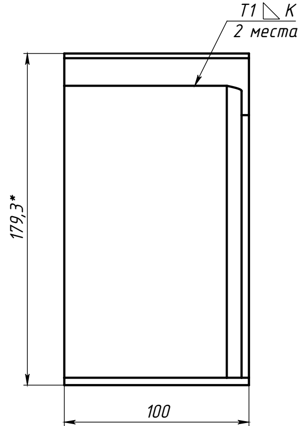
Поз.3 (Ложемент)
