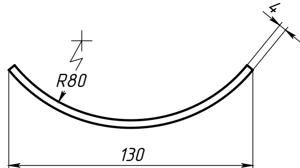
Поз.3 (Ложемент)
